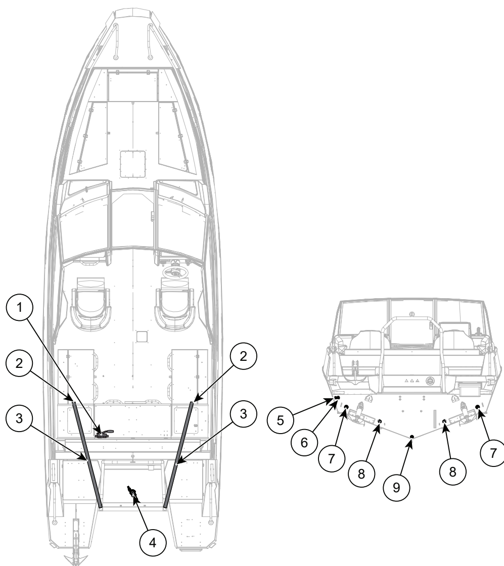
Kuva 9.1 Buster Magnum/SuperMagnum pilssipumput ja tyhjennys
