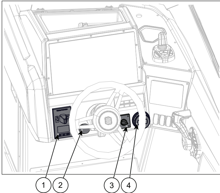
Kuva 5.2 Ohjauspisteen hallintalaitteet, kun varusteena on integroitu keulapotkuri
