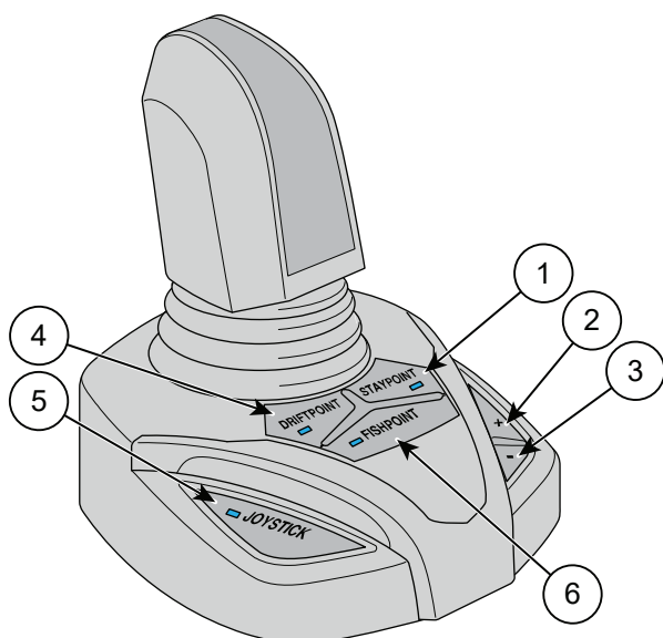
Kuva 5.5 Joystick-ohjain ja toimintopainikkeet
