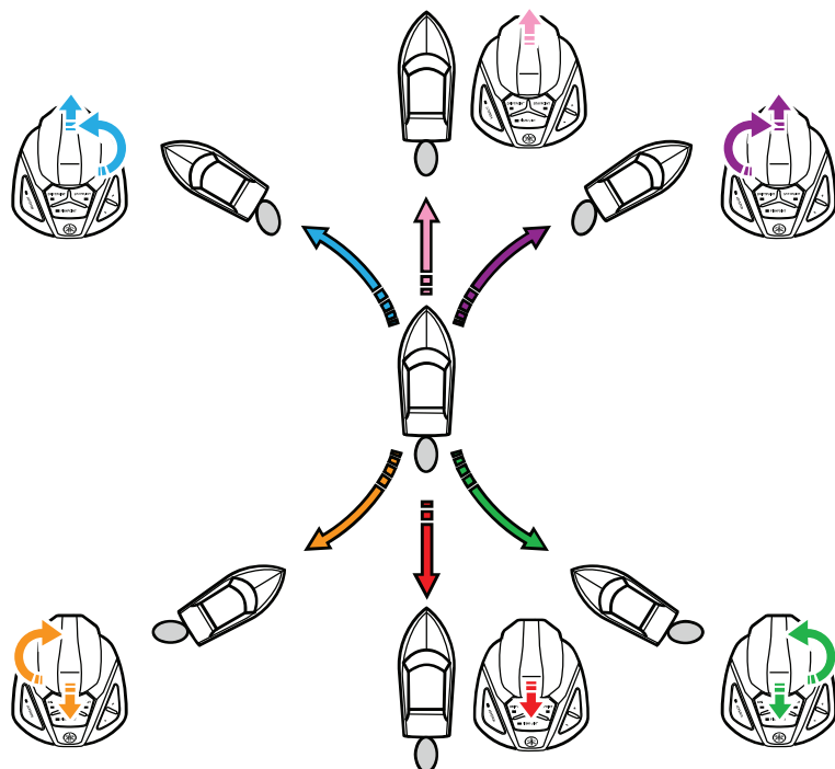
Kuva 5.6 Joystick-ohjaimen käyttö yksimoottorisessa veneessä
