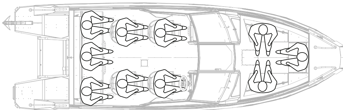
Kuva 4.3 SuperMagnum performance pack -istuimet enintään kymmenelle (10) matkustajalle
