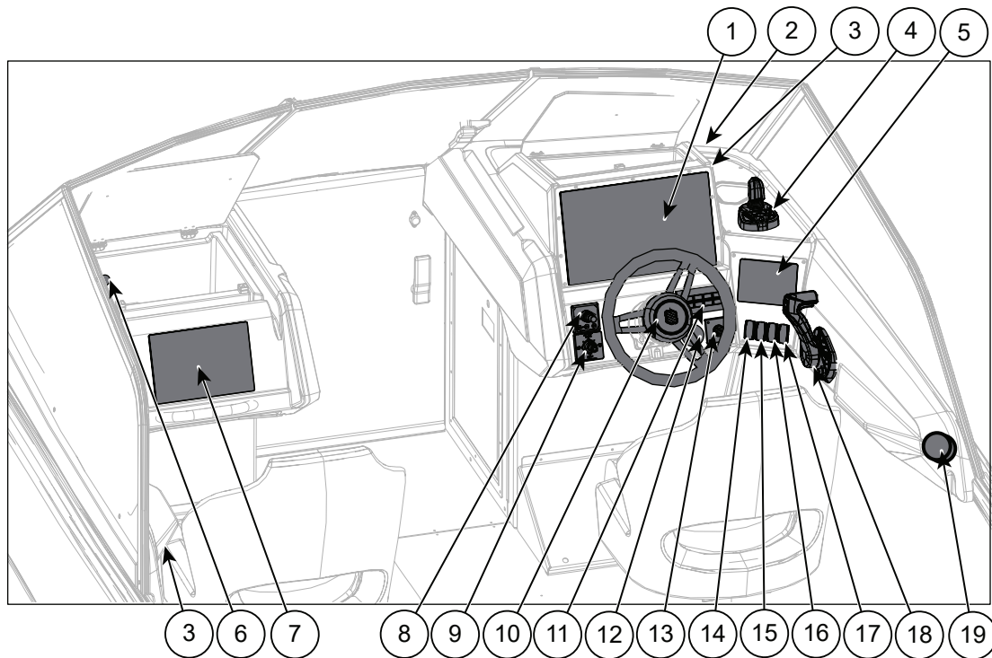
Kuva 5.1 Buster Magnum/SuperMagnum ohjauspisteen hallintalaitteet
