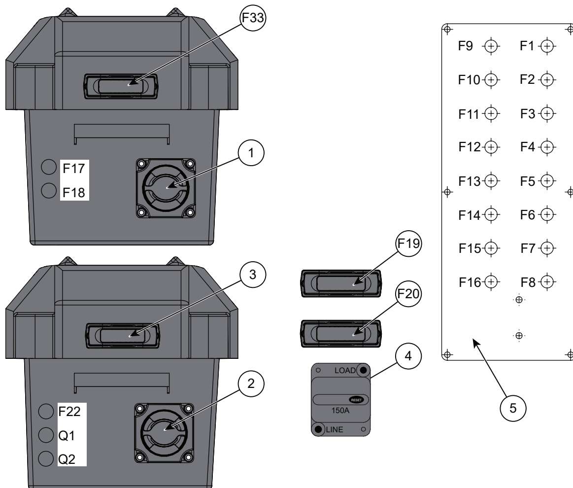
Kuva 8.1 Buster Magnum/SuperMagnum päävirtakytkimet ja sulakepaneelit
