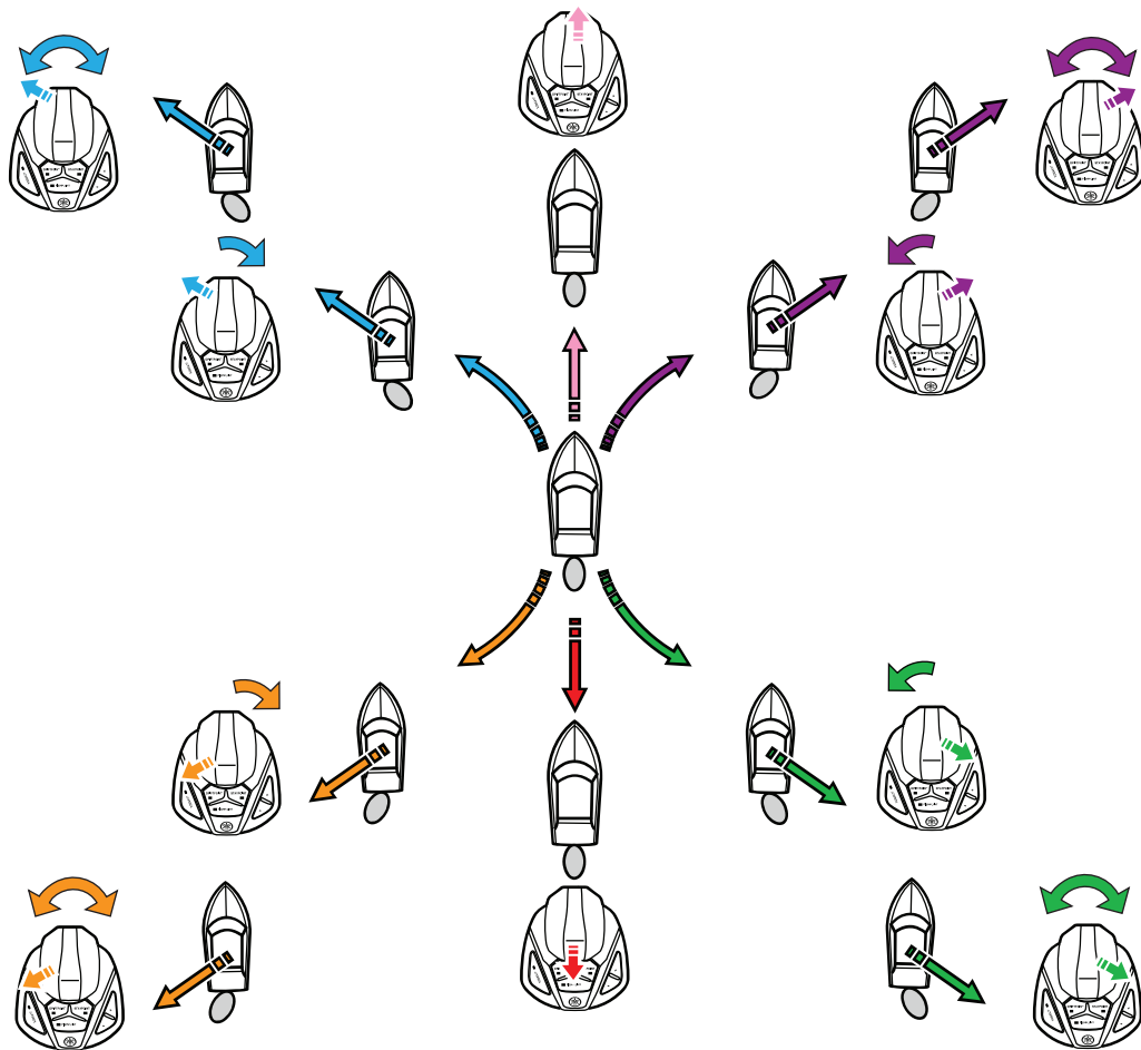
Kuva 5.9 Joystick-ohjaimen käyttö integroidun keulapotkurin hallinnan kanssa
