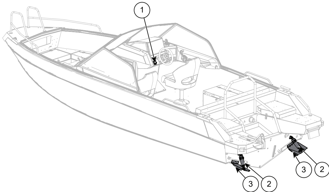
Kuva 5.10 Buster Magnum/SuperMagnum trimmijärjestelmä
