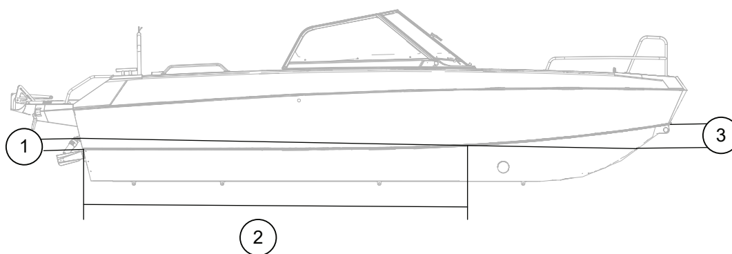
Kuva 3.1 Buster Magnum/SuperMagnum anti-fouling-maalialue
