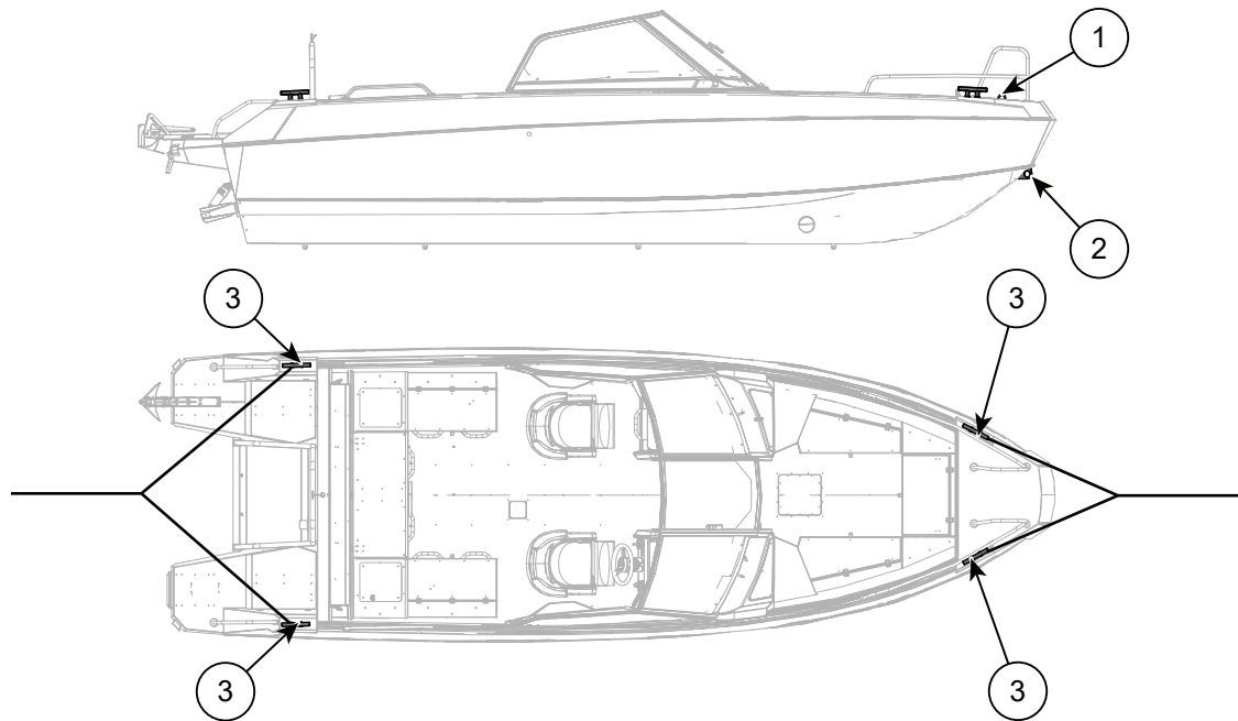
Kuva 5.11 Buster Magnum/SuperMagnum kiinnitys- ja hinauspisteet
