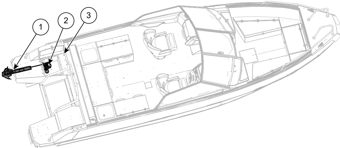
Kuva 10.1 Buster Magnum/SuperMagnum ankkurivinssi
