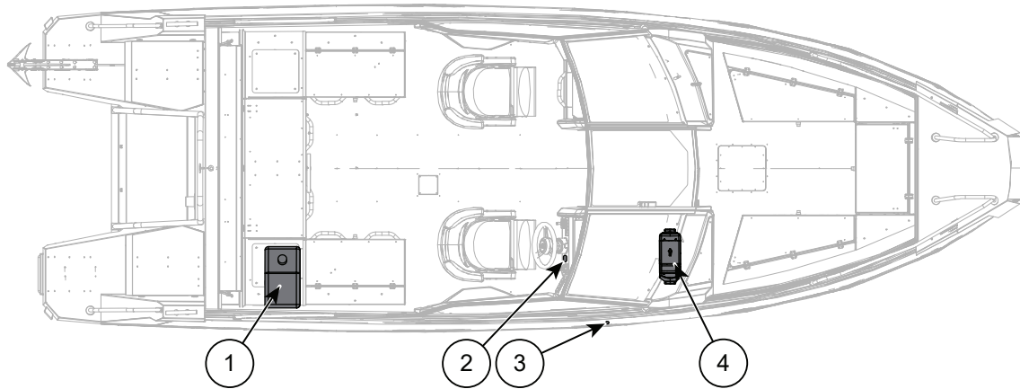
Kuva 6.2 Buster Magnum/SuperMagnum lämmitysjärjestelmä
