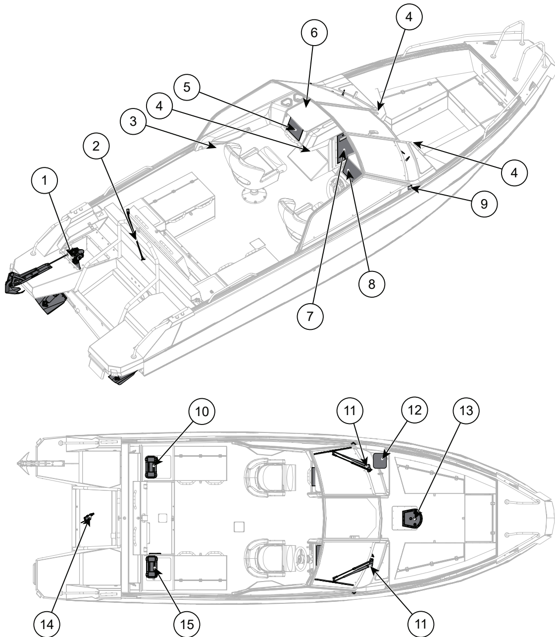
Kuva 8.3 Buster Magnum/SuperMagnum sähkölaitteet
